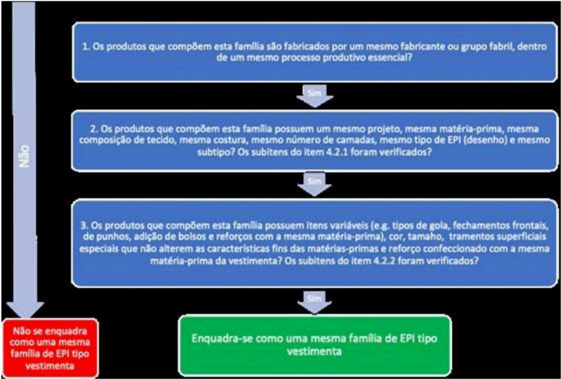
Figura 1 - Definição de família de EPI tipo vestimenta
